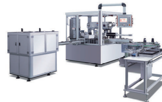
단색 파우더 전자동 프레스 ZPRESS-8D
