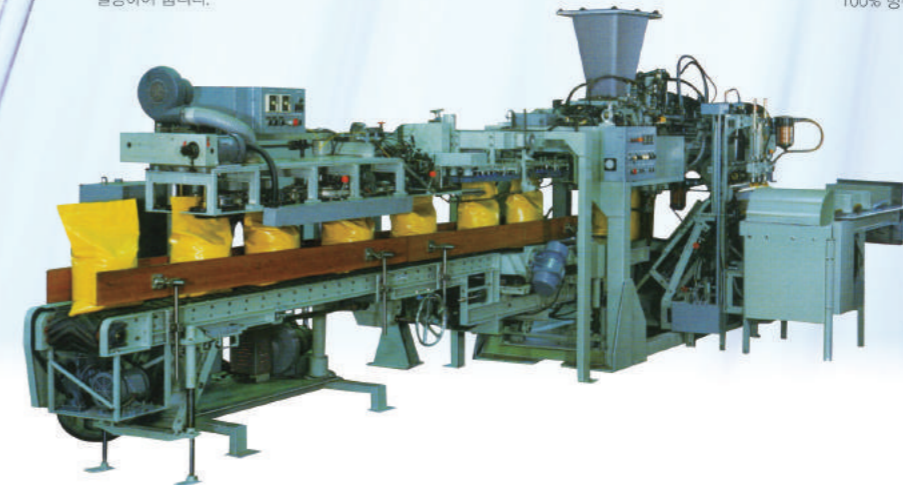
PBC-3W (Pinch Bag Sealing) 1. 백상입에서 실링봉함까지 완전 자동. 2. 내용물, 백사양에 따라서 7가지의 표준모델이 준비되어있음. 3. 뜨거운 공기로 핫멜트를 녹인 후 프레스롤로 완전히 백을 압착시킨다. 더블핀치의 경우 내용물을 먼저나 숨기로부터 보호하기위해 내부 PE를 실링하여 줍니다.
